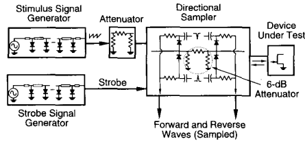
Fig. 3. NWA IC block diagram.
